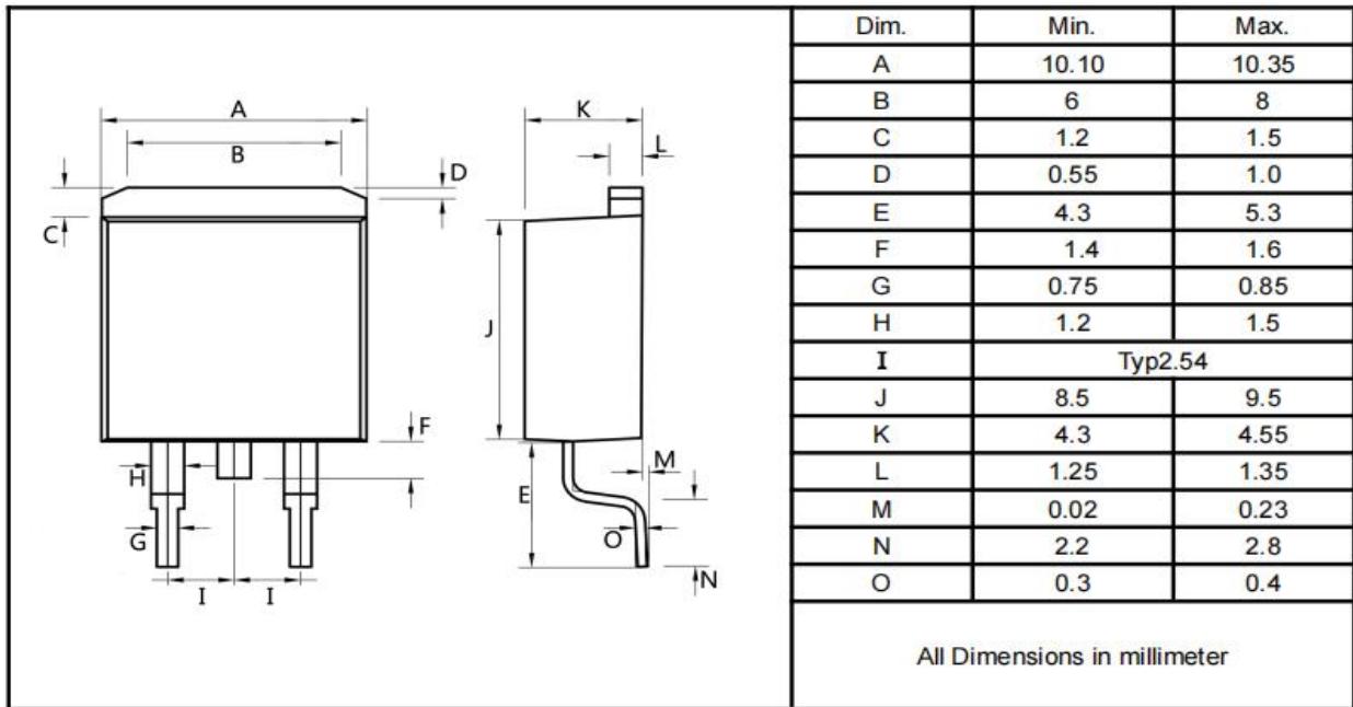
TO-263
